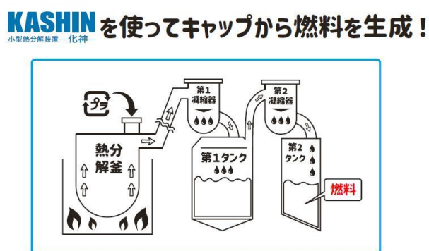
参考：(4) プラごみ集めて船を走らせよう！で軽油生成に使用する小型熱分解装置
